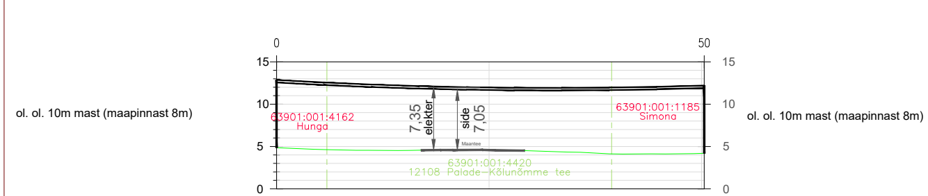
12108 Palade-Kõlunõmme tee õhuliini visangu ristlõige2
