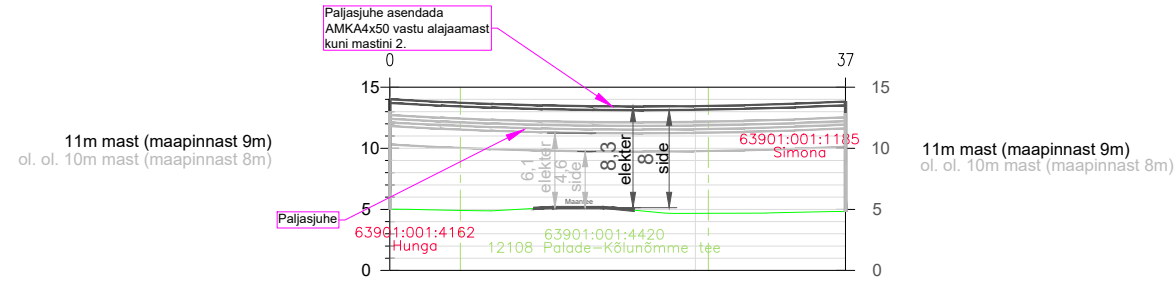
12108 Palade-Kõlunõmme tee õhuliini visangu ristlõige1
